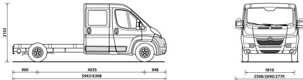
Šasija s produženom kabinom L3/L4
