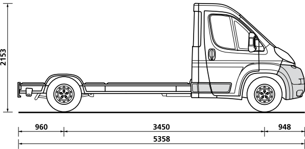
Šasija s niskim podom L2
