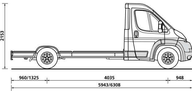
Šasija s niskim podom L3/L4
