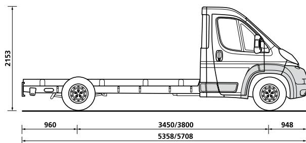
Šasija s kabinom L2/L2S
