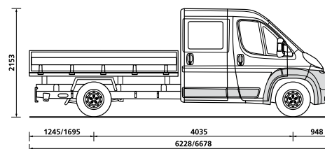
Platforma s produženom kabinom L3/L4
