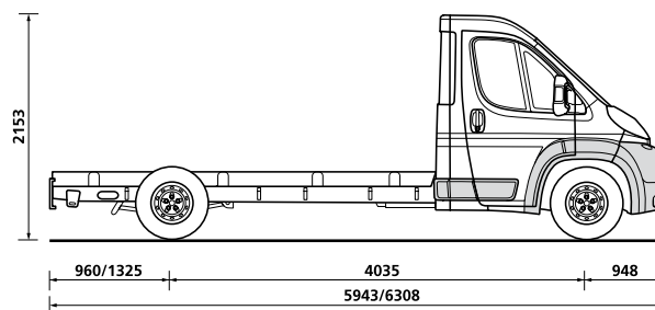
Šasija s kabinom L3/L4
